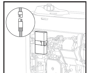
Anschließen der Plus- und Minuskabel
