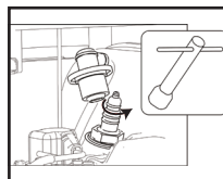
De bougie verwijderen
